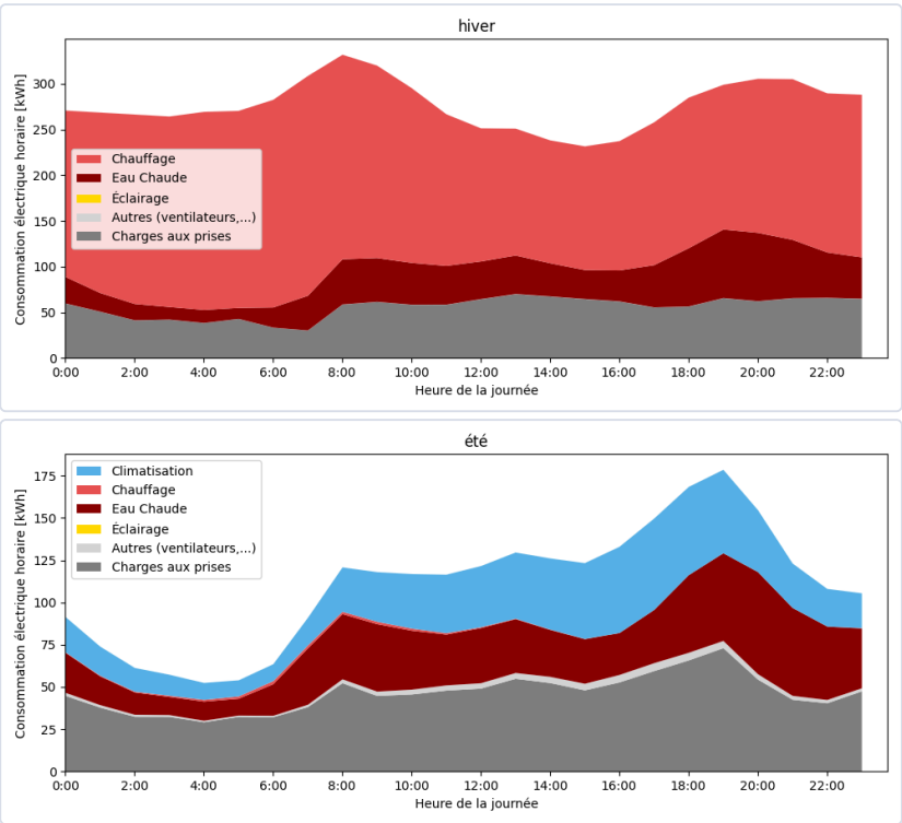
Profil de consommation journalière moyen des jours d'hiver et d'été, montrant la contribution du chauffage, de l'éclairage, de l'eau chaude sanitaire, des charges aux prises et des systèmes auxiliaires au cours d'une journée hivernale ou estivale moyenne.
